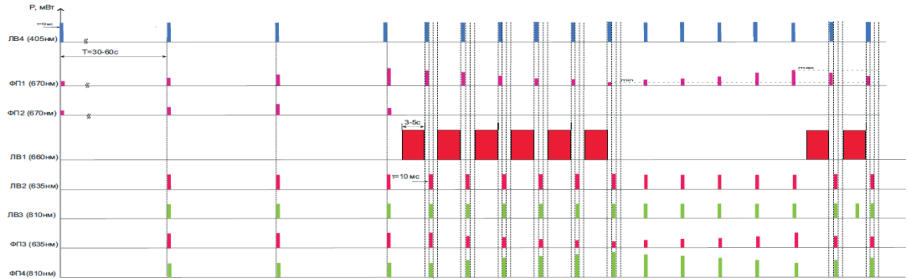
Рисунок 9 – Часові діаграми одного з можливих варіантів функціонування оптико-електронного приладу
