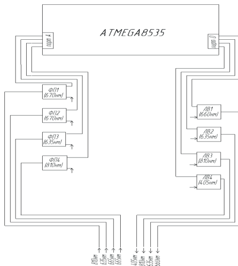
Рисунок 8 – Функціональна схема реалізації оптико-електронного приладу для оксиметрично-корегової фотодинамічної терапії пухлин
