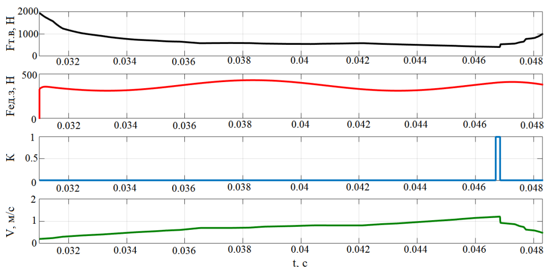
Рисунок 4.8 – Результати моделювання комп'ютерної моделі виявлення та попередження зносу контактної системи при ввімкненні вакуумного вимикача
