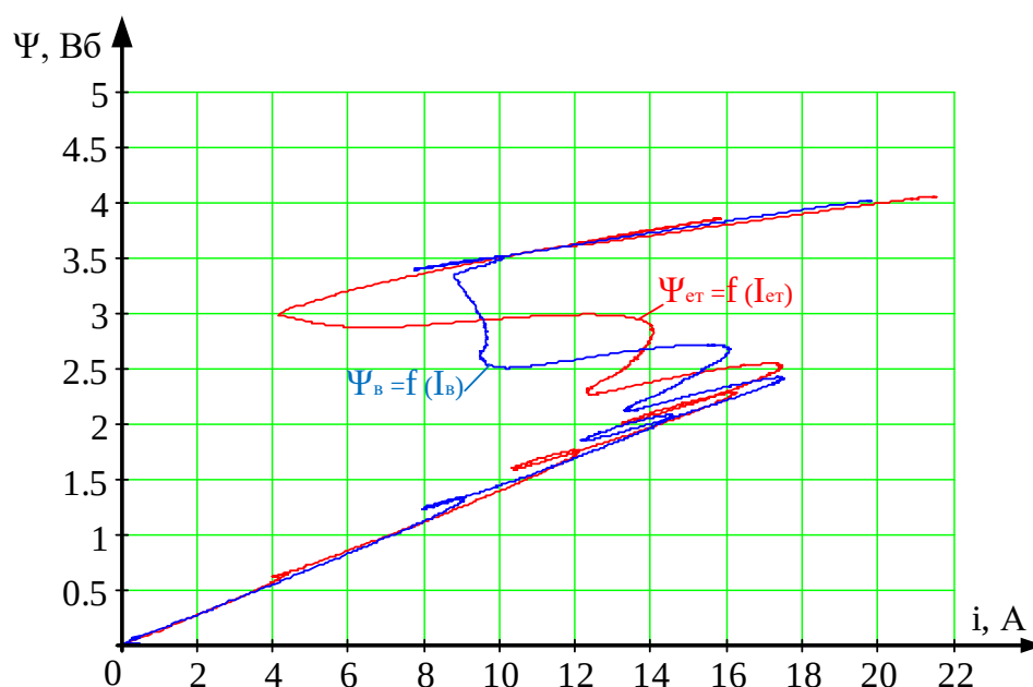
Рисунок 4.17 – Порівняння вебер-амперних характеристик справного \Psi_{ет} = f(I_{ет}) та з дефектом \Psi_{в} = f(I_{в}) електромагнітного привода вакуумного вимикача для обмотки вимкнення
