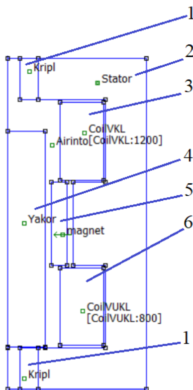
Рисунок 4.2 – Розрахункова модель магнітної системи електромагнітного приводу вакуумного вимикача у програмі FEMM
