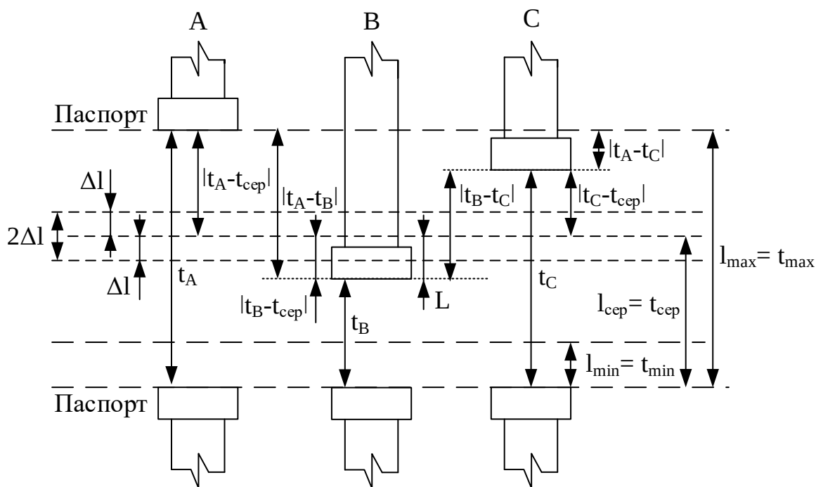
Рисунок 2.3 – Часові діаграми неузгодження ввімкнення контактної системи полюсів вимикача
