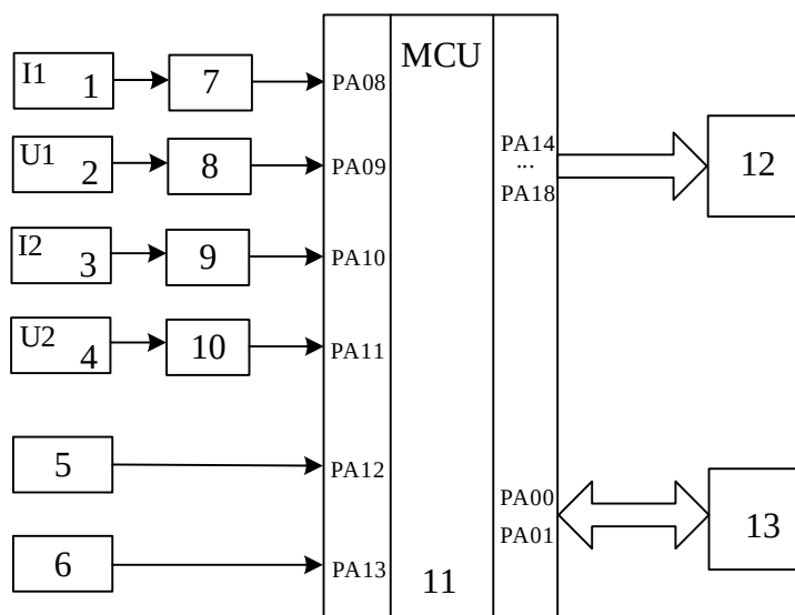
Рисунок 3.1 – Структурна схема блока діагностування електромагнітного привоу вакуумного вимикача
