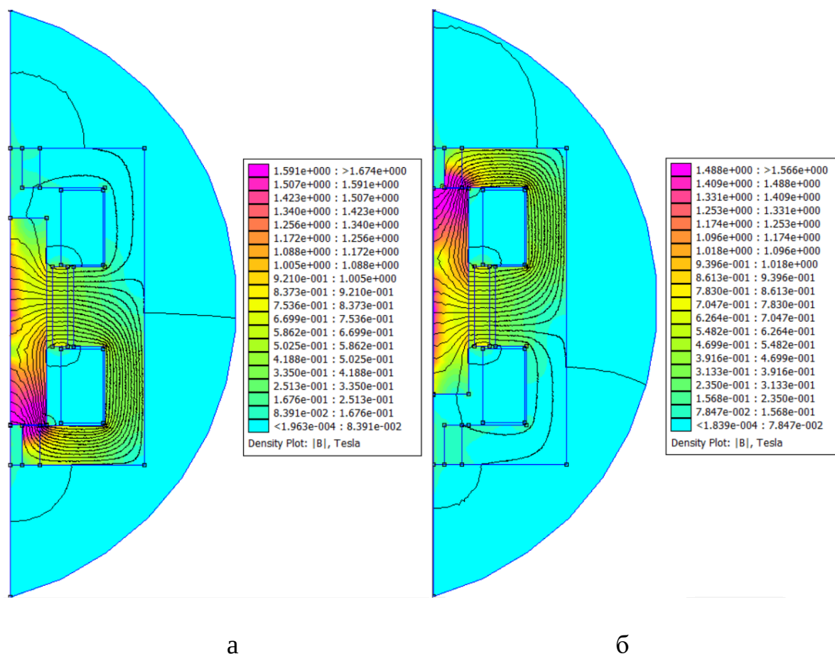
Рисунок 4.3 – Розподіл магнітного поля в електромагніті вакуумного вимикача у крайніх положеннях: а – електромагніт у вимкненому положенні; б – електромагніт у ввімкненому положенні
