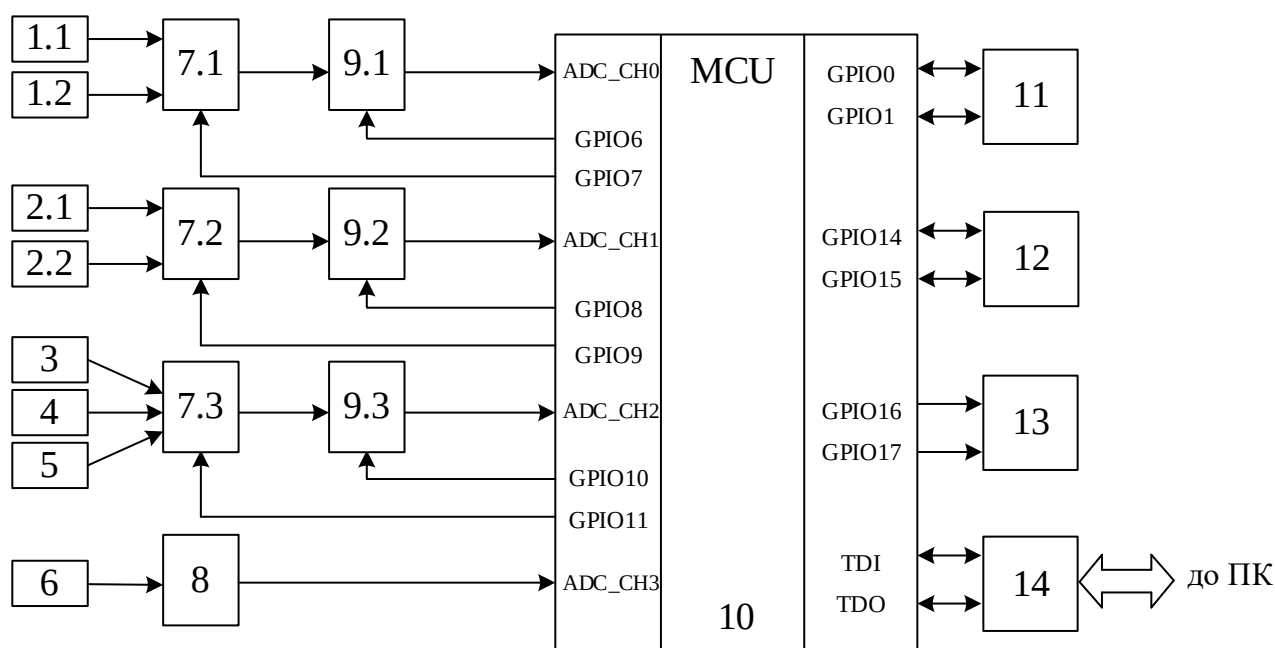
Рисунок 3.9 – Структурна схема мікропроцесорного пристрою системи виявлення зносу контактної системи вакуумного вимикача
