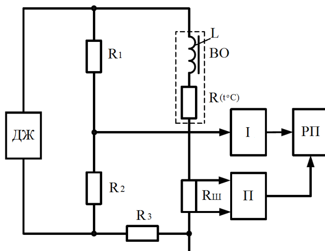
Рисунок 1.4 – Структурна схема “безсенсорного” пристрою випробування електромагніту
