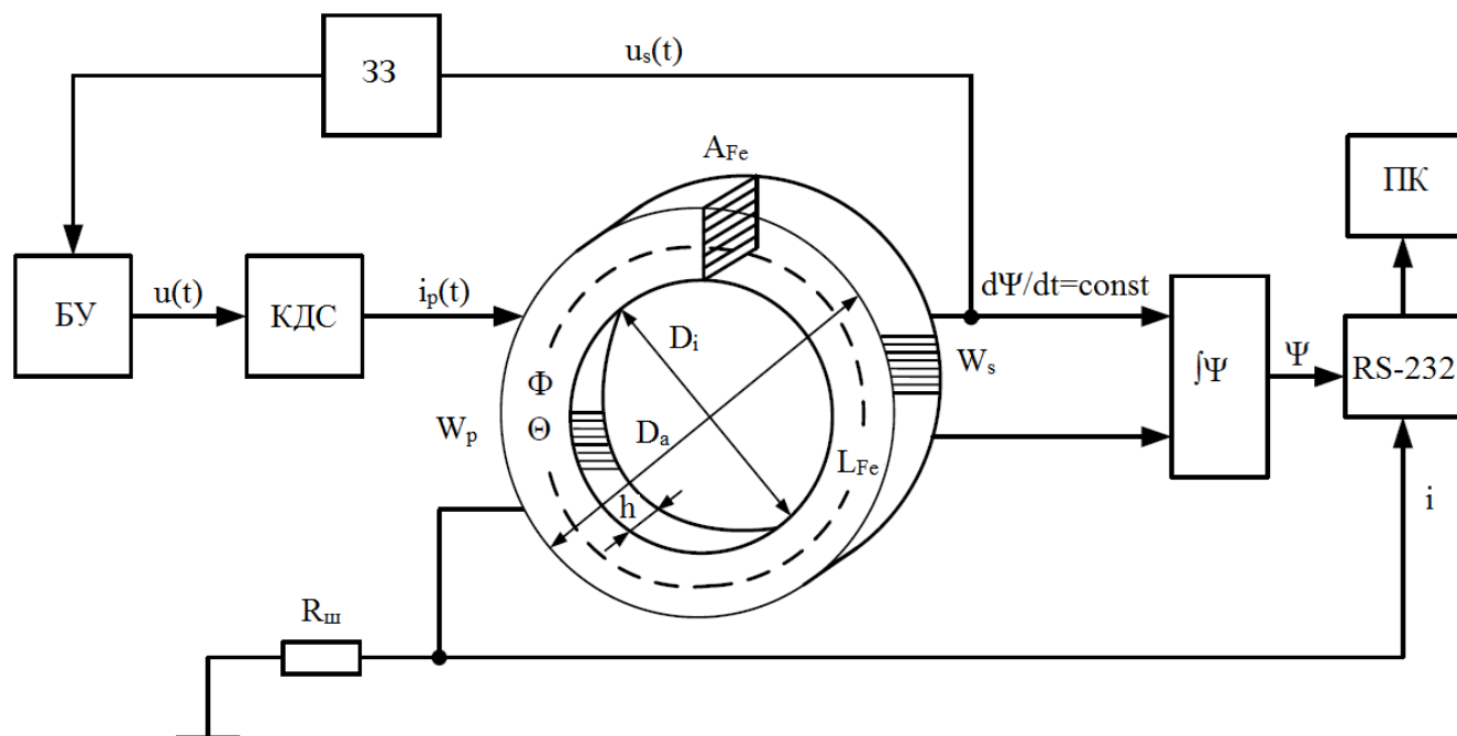
Рисунок 1.5 – Функціональна схема ABC MagHyst
