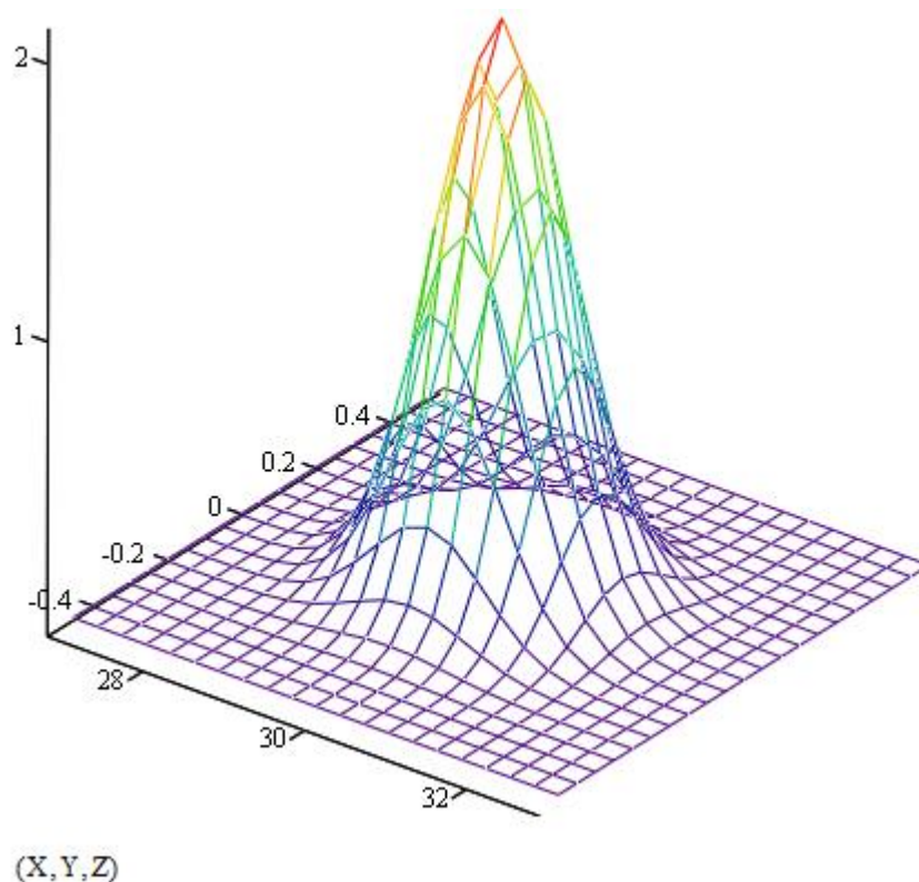
Рисунок 4.19 – Графічне представлення сумісного закону розподілу
