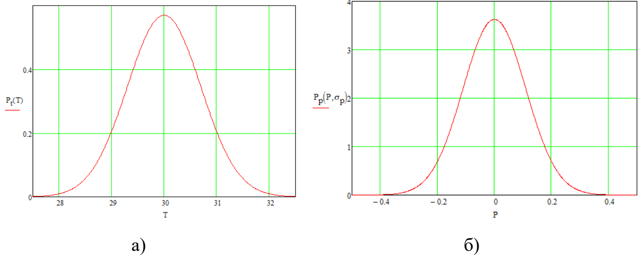
Рисунок 4.18 – Графічне представлення законів розподілу: а) вимірюваного часу неодночасності комутації; б) похибки вимірювання часу неодночасності комутації
