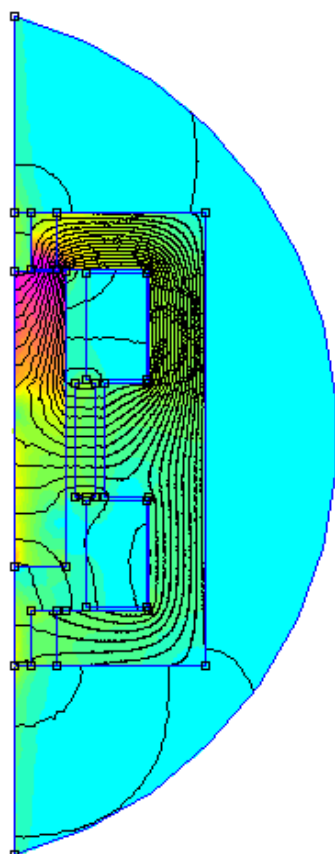
Розрахунок параметрів електричного кола для блока CoilVUKL
