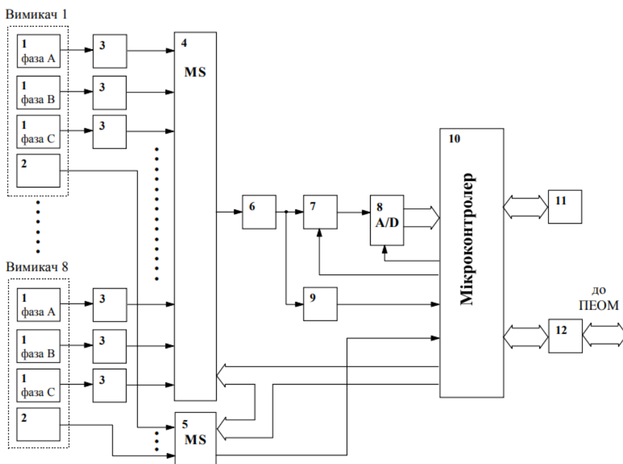
Рисунок 1.8 – Структурна схема базового блока системи діагностування вимикачів
