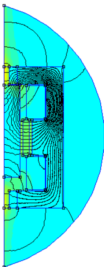
Розрахунок параметрів електричного кола для блока CoilVKL
