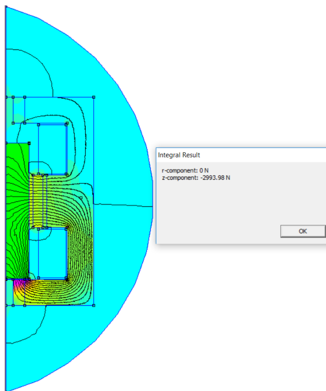
Рисунок 4.4 – Розрахунок сили утримання якоря електромагніта у вимкненому положенні методом інтеграла тензора Максвелла
