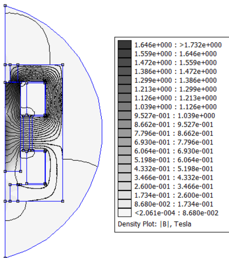
Картина поля ліній потоку електромагнітного приводу
