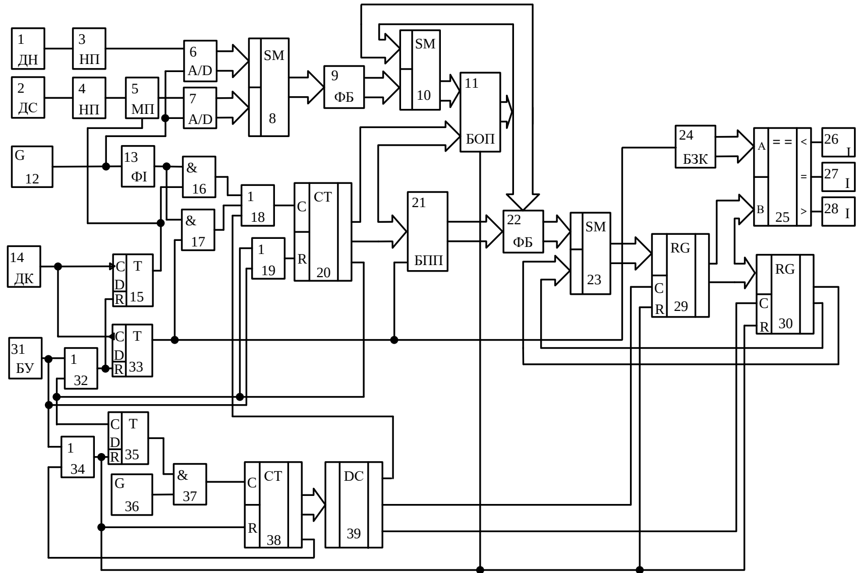
Рисунок 3.3 – Схема пристрою для діагностування електричного приводу вимикача
