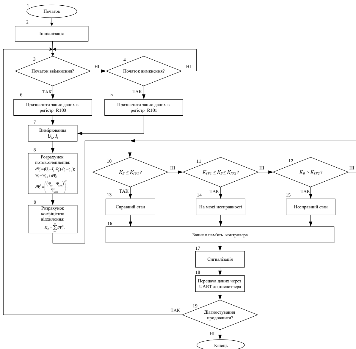
Рисунок 3.2 – Алгоритм роботи мікропроцесорного пристрою діагностування електромагнітного приводу вакуумного вимикача
