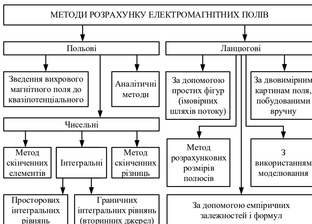
Рисунок 4.1 – Основні методи розрахунку електромагнітних полів
