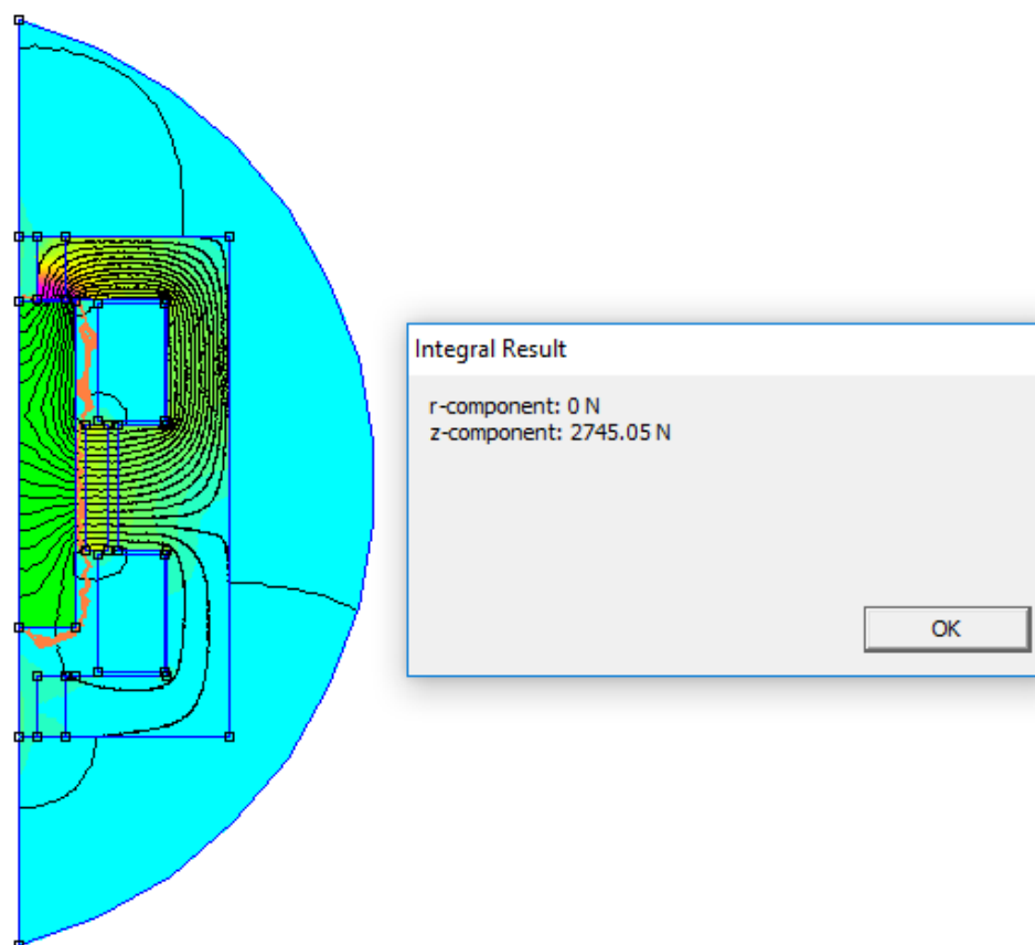
Розрахунок сили утримання приводу методом інтеграла тензора Максвелла
