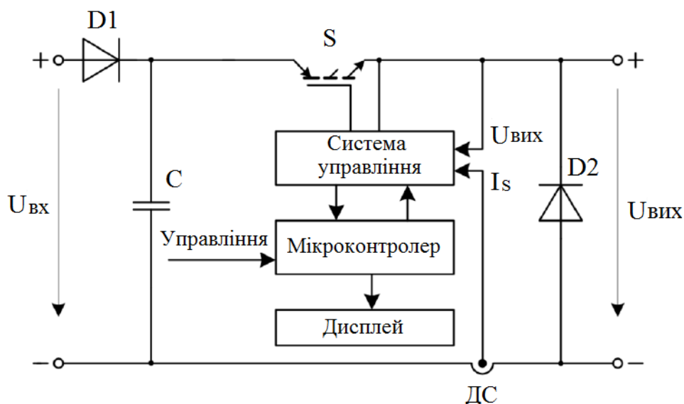
Рисунок 1.3 – Функціональна схема пристрою контролю роботи приводу вимикача
