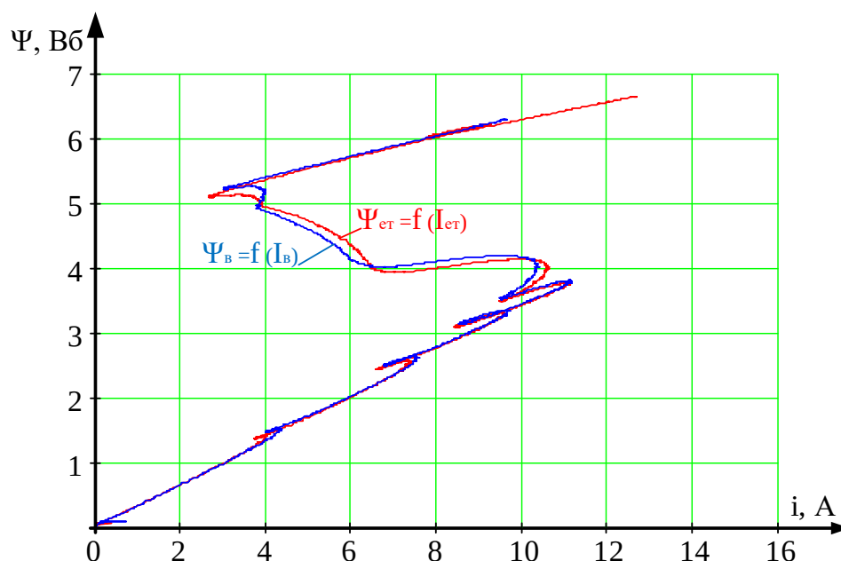
Рисунок 4.16 – Порівняння вебер-амперних характеристик справного \Psi_{ет} = f(I_{ет}) та з дефектом \Psi_{в} = f(I_{в}) електромагнітного привода вакуумного вимикача для обмотки ввімкнення
