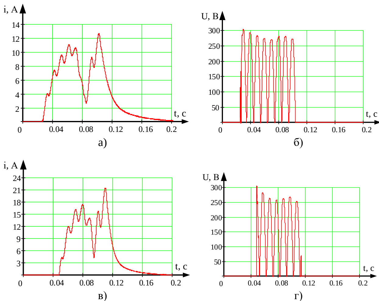
Рисунок 4.12 – Графіки струму та напруги при вмиканні та вимиканні вимикача:
