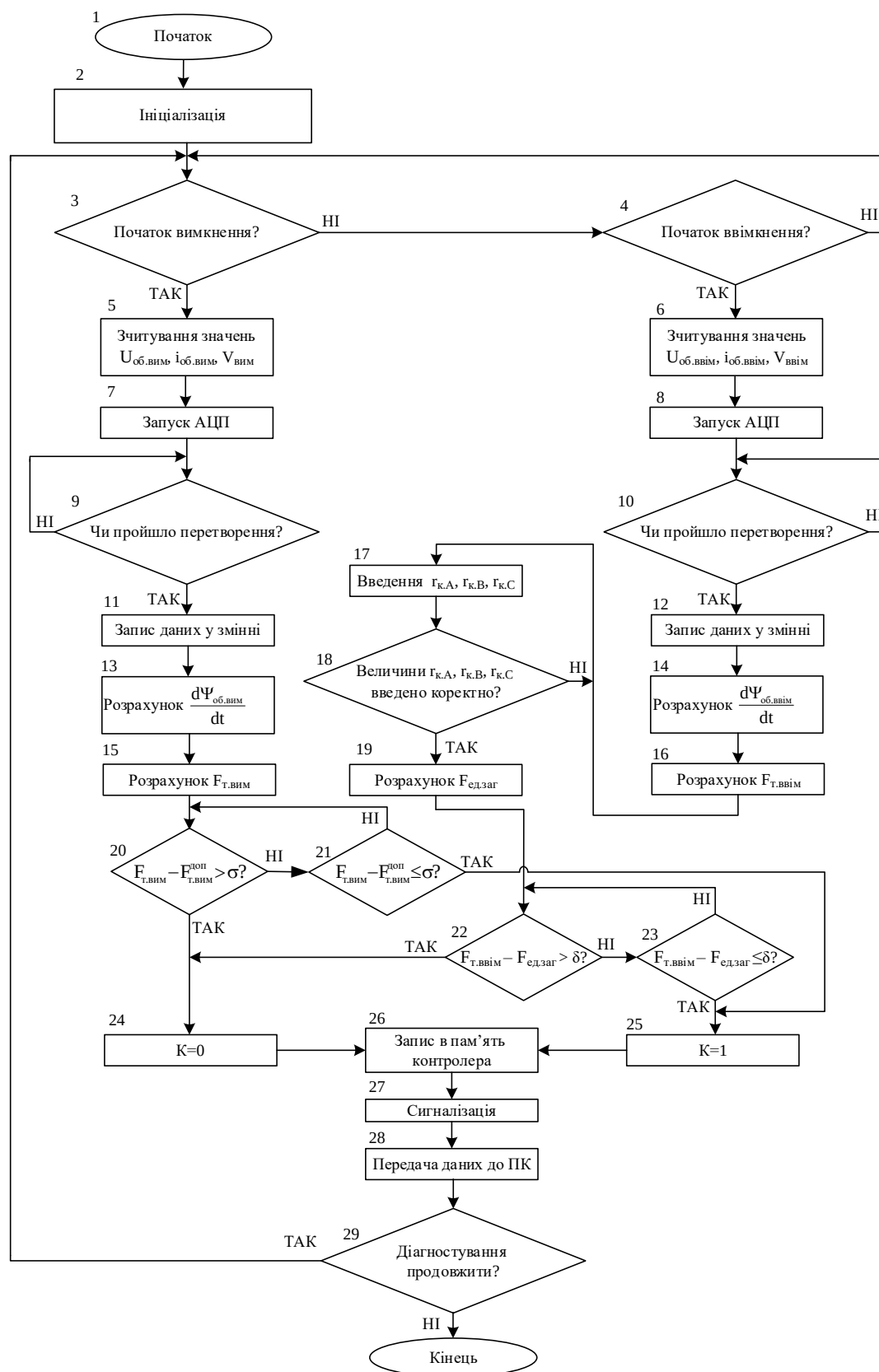
Рисунок 3.10 – Узагальнений алгоритм роботи мікропроцесорного пристрою
