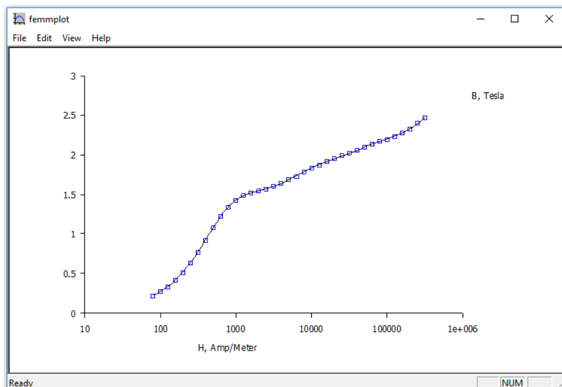
Логарифмічний графік кривої намагнічення для блока Stator
