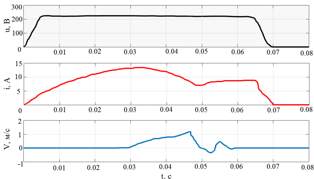
Рисунок 4.7 – Результати моделювання електричних параметрів (напруги і струму обмотки ввімкнення) та механічних (швидкості руху якоря) електромагнітного приводу при ввімкненні вакуумного вимикача
