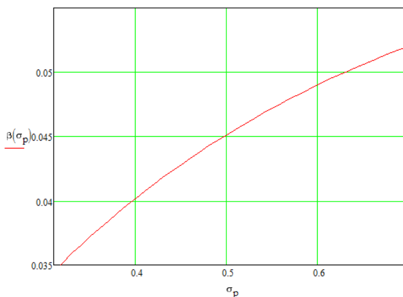
Рисунок 4.21 – Номограма визначення помилки другого роду
