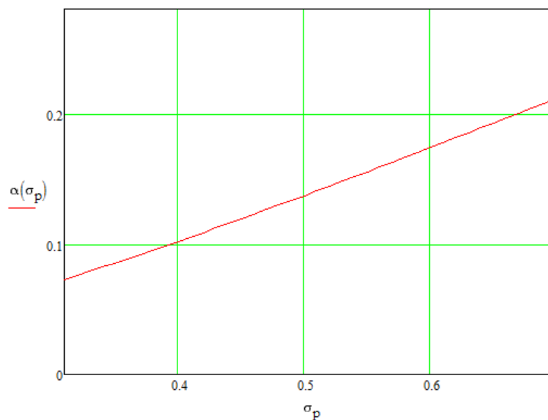
Рисунок 4.20 – Номограма визначення помилки першого роду
