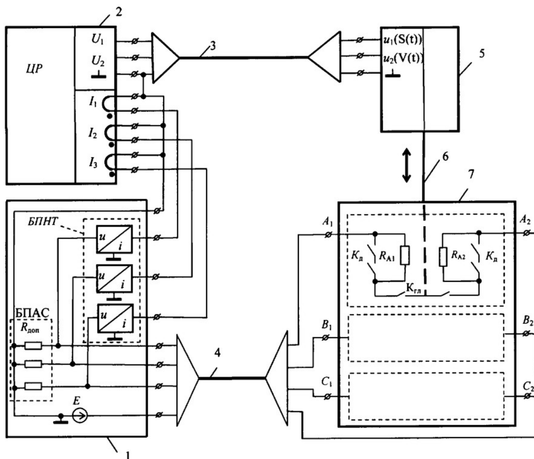
Рисунок 1.7 – Схема пристрою прискореного контролю характеристик високовольтних вимикачів
