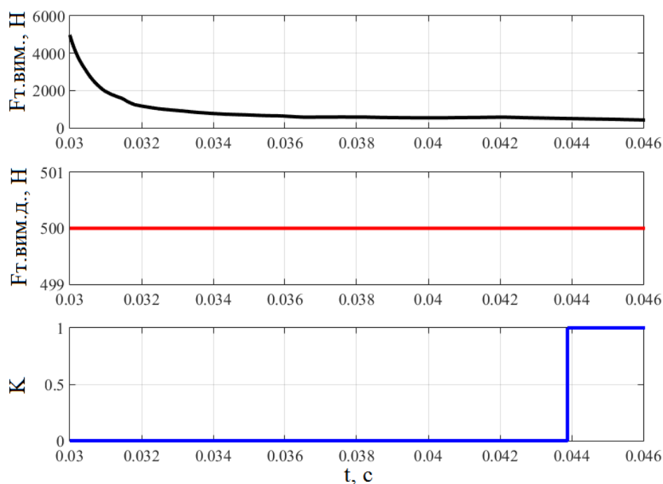
Рисунок 4.10 – Результати моделювання комп'ютерної моделі виявлення та попередження зносу контактної системи при вимкненні вакуумного вимикача
